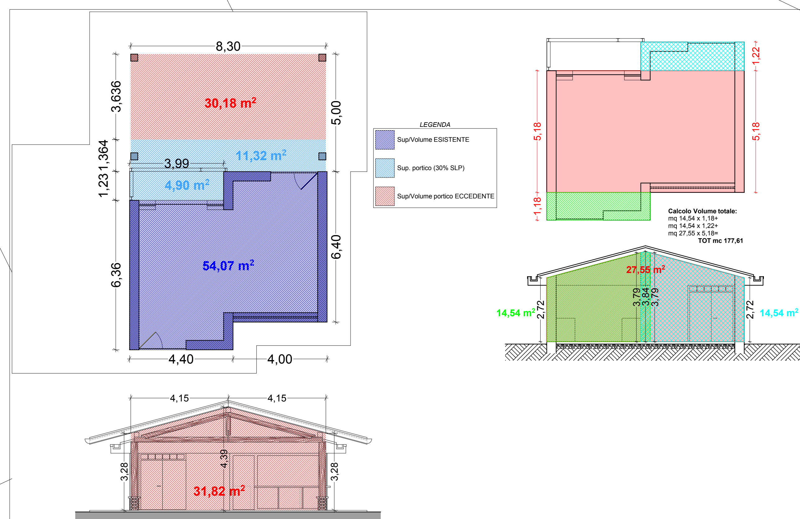
SCHEMA CALCOLO SUPERFICI E VOLUME: PUNTO RISTORO/BAR - scala 1:100 -
