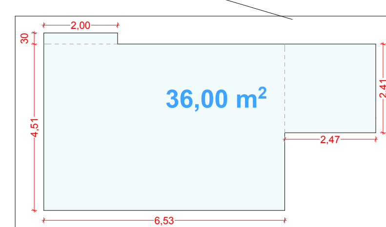
SCHEMA CALCOLO SUPERFICIE: SERVIZI IGIENICI - scala 1:100 -
