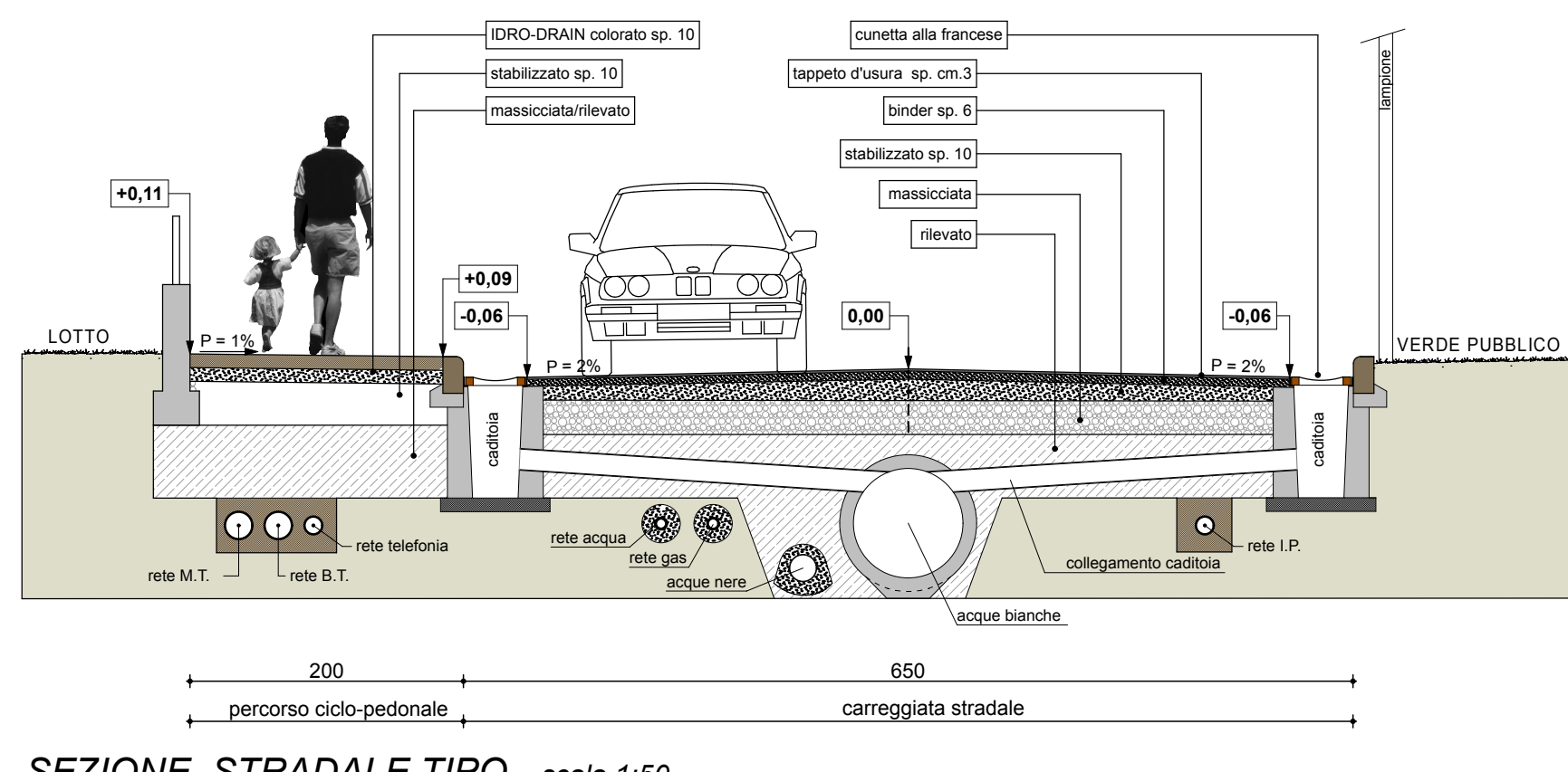
SEZIONE STRADALE TIPO - scala 1:50
