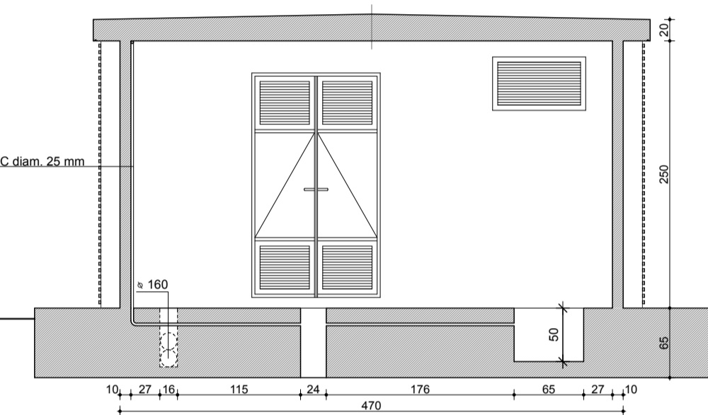
SEZIONE A-A
