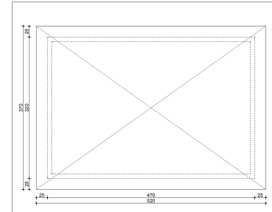
COPERTURA
