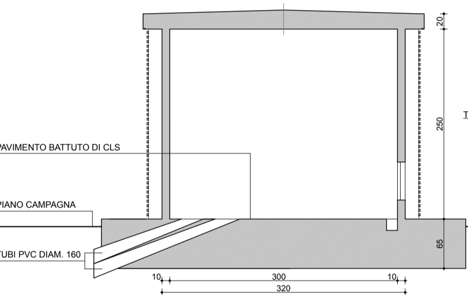
SEZIONE B-B
