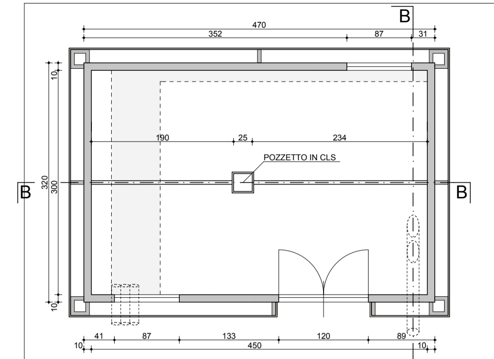
PIANTA
