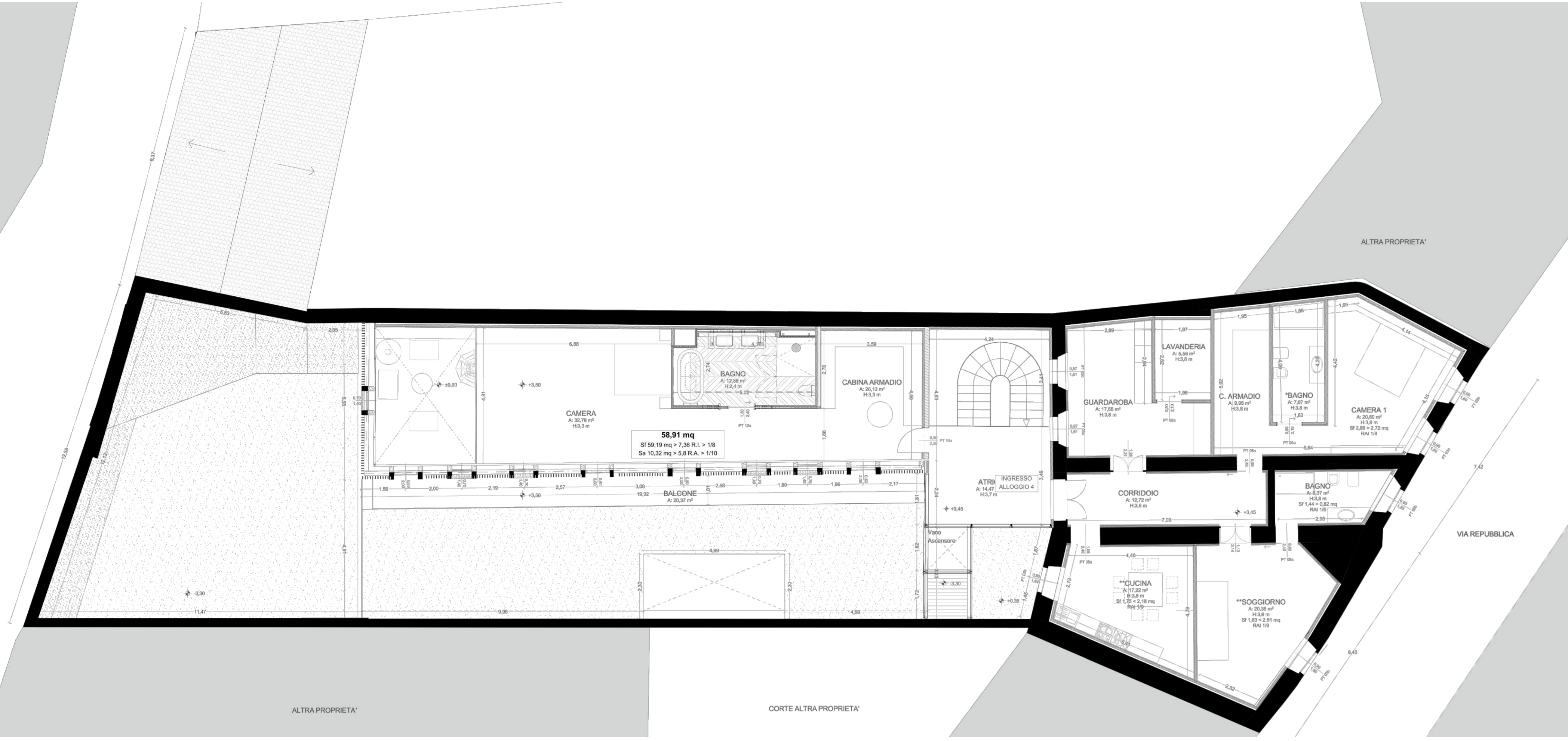
Pianta Piano Primo Stato Autorizzato
