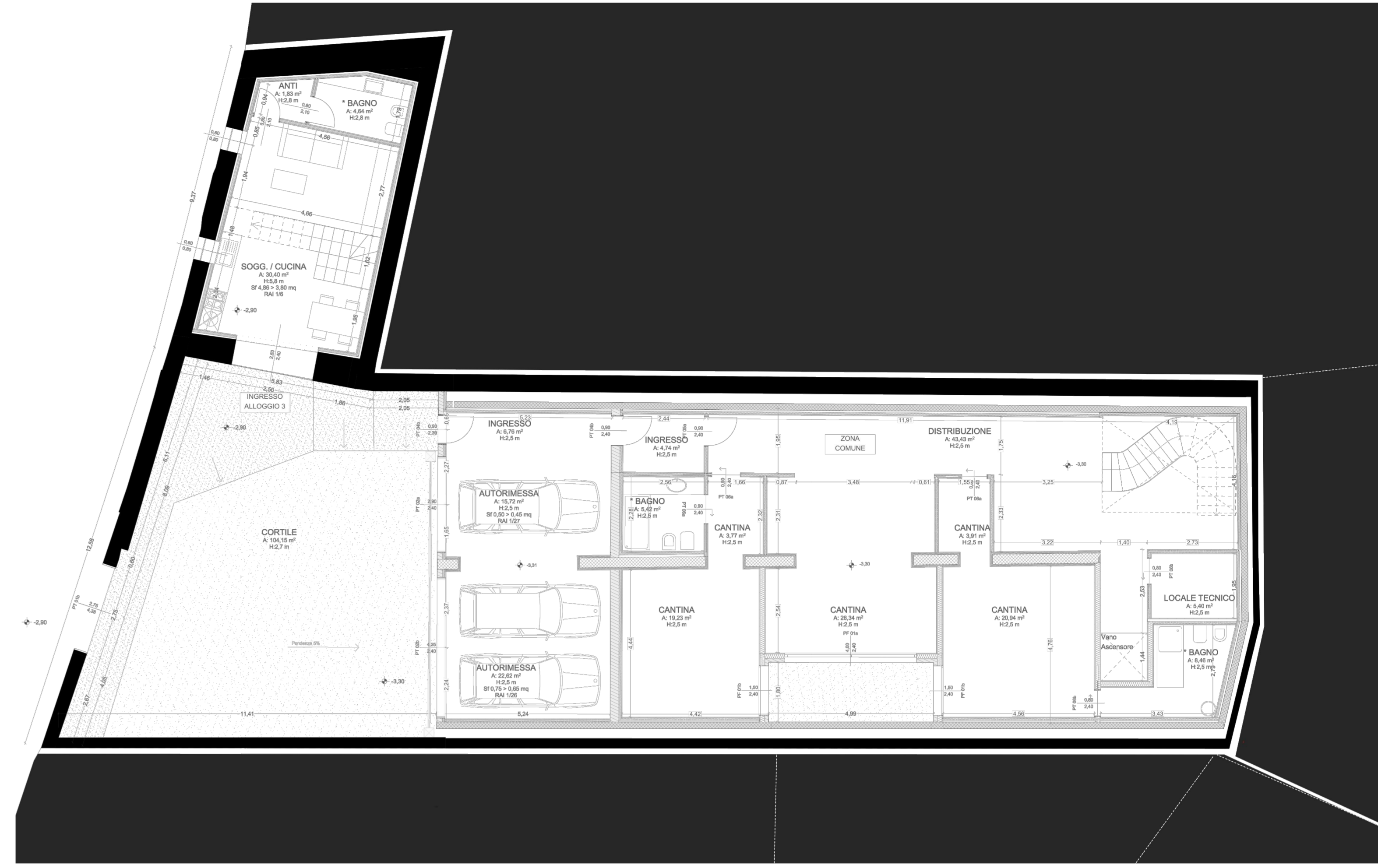
Pianta Piano Interrato Stato Autorizzato
