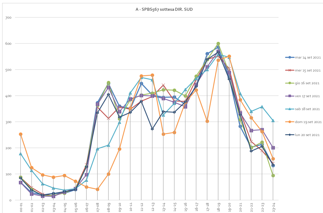
Figura 16 – Postazione A – SS32, andamento giornaliero/orario dei flussi di traffico
