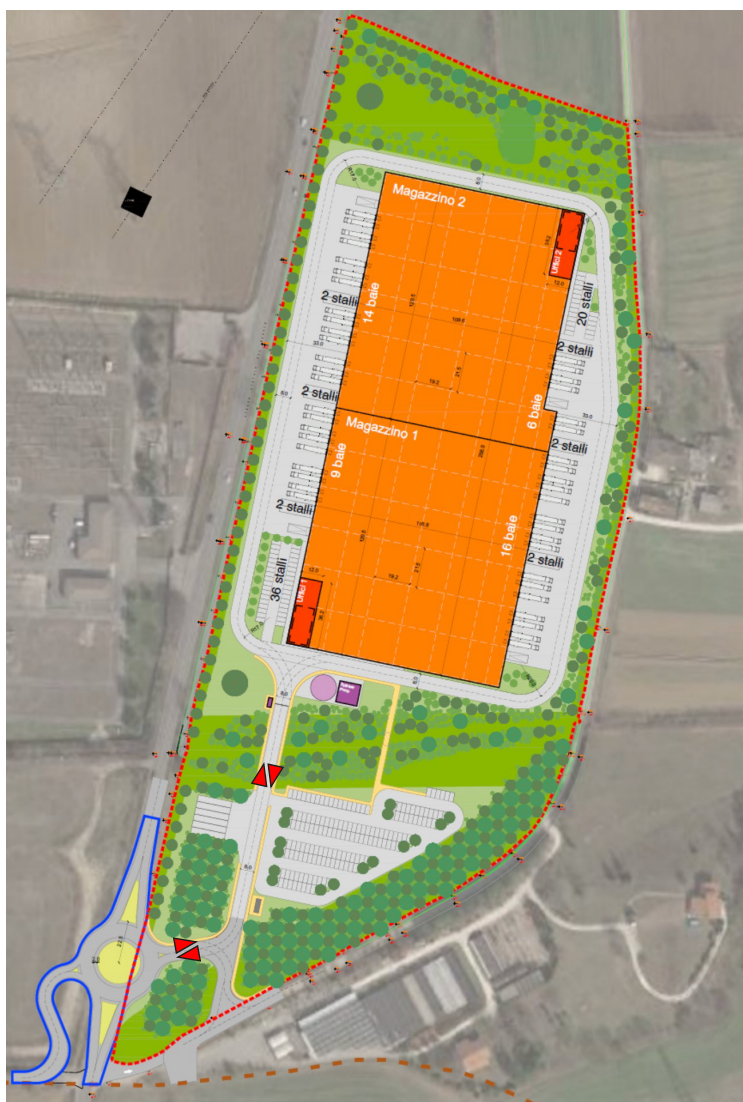
Figura 28 – Planimetria di progetto dell'intervento e localizzazione degli accessi
