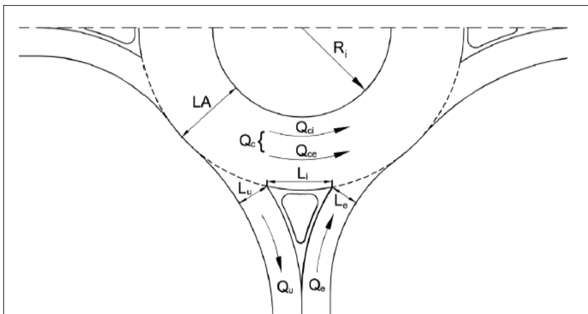
Figura 32 – Grandezze geometriche e funzionali utilizzate dal software Girabase
