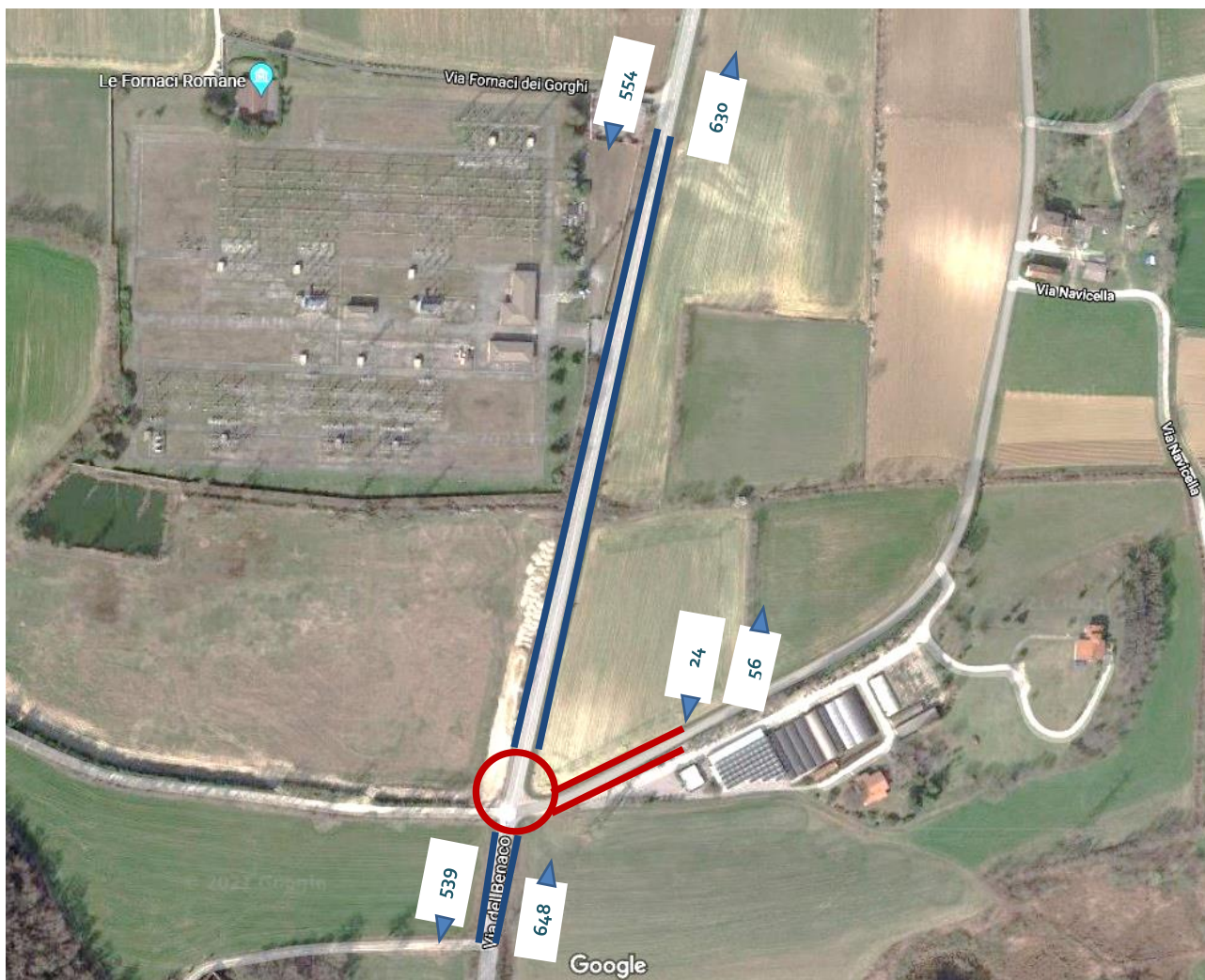
Figura 30 – Scenario di progetto, flussi veicolari attesi nell'ora di punta del mattino (vph eq)
