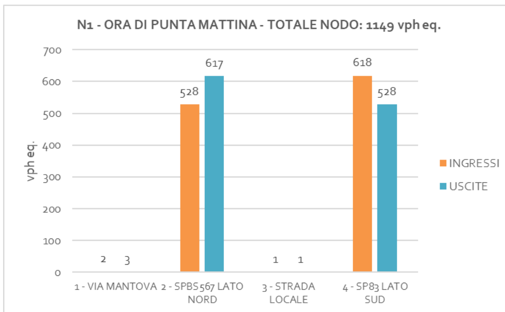
Figura 17 – Nodo N1, valori di sezione sui rami afferenti al nodo nell’ora di punta del mattino (vph eq)
