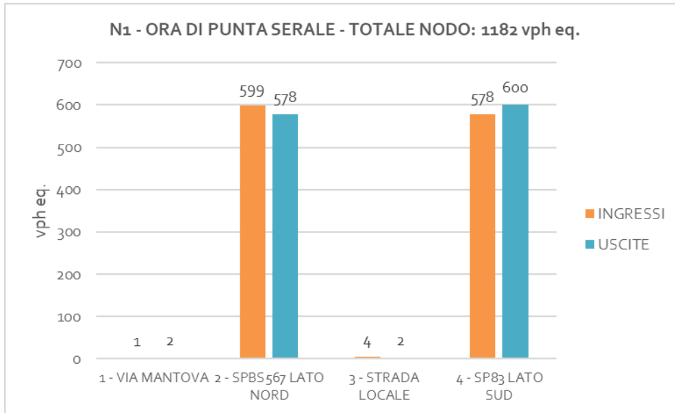
Figura 18 – Nodo N 1 , valori di sezione sui rami afferenti al nodo nell'ora di punta serale (vph eq)
