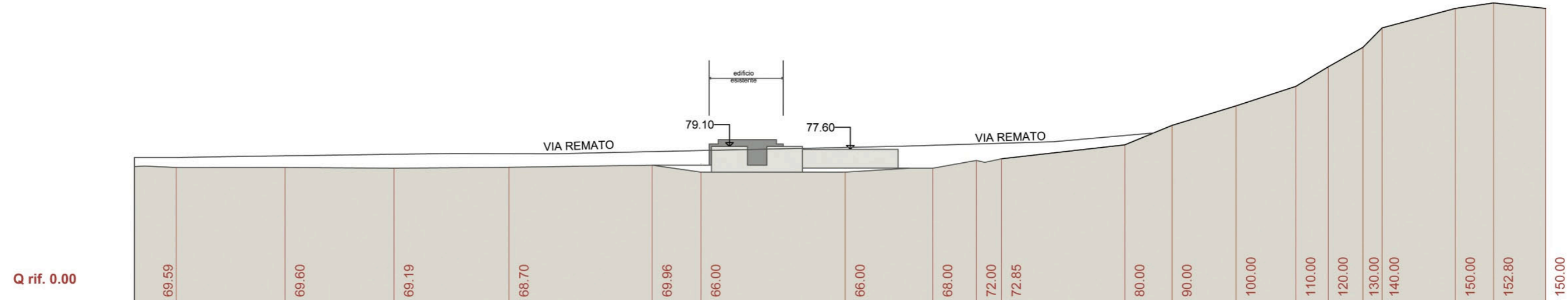
PROFILO X-X 1:2000
