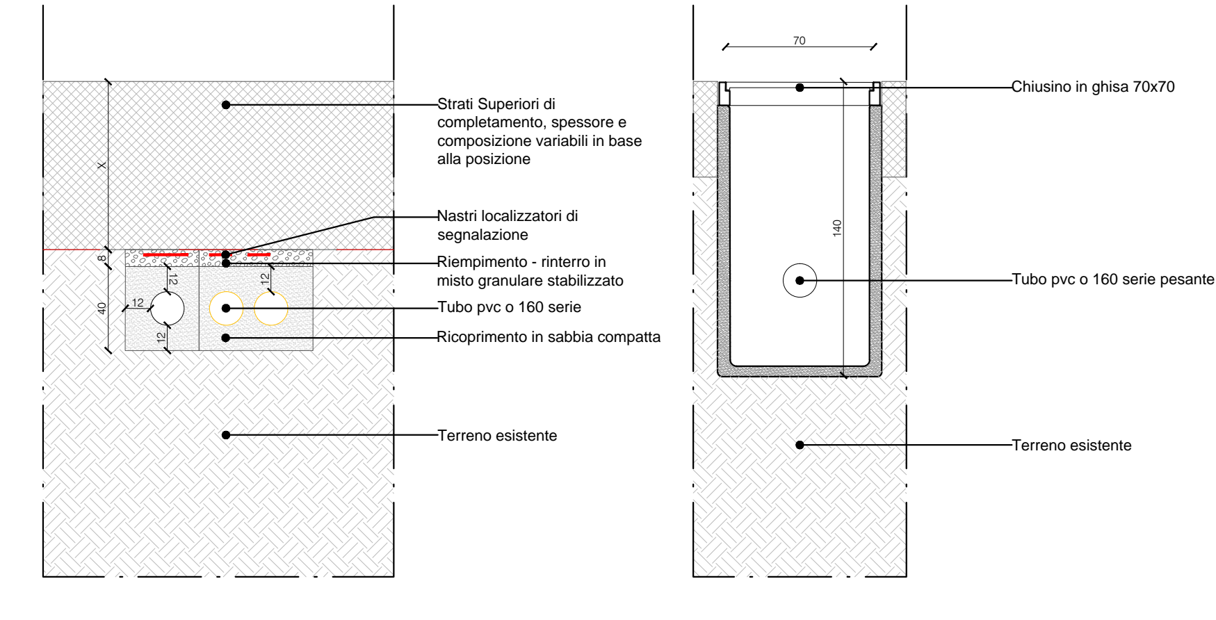
Dettaglio costruttivo rete idrica (scala 1:20)
