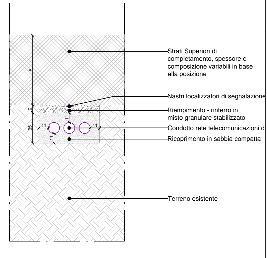
Dettaglio costruttivo rete telecomunicazioni (scala 1:20)
