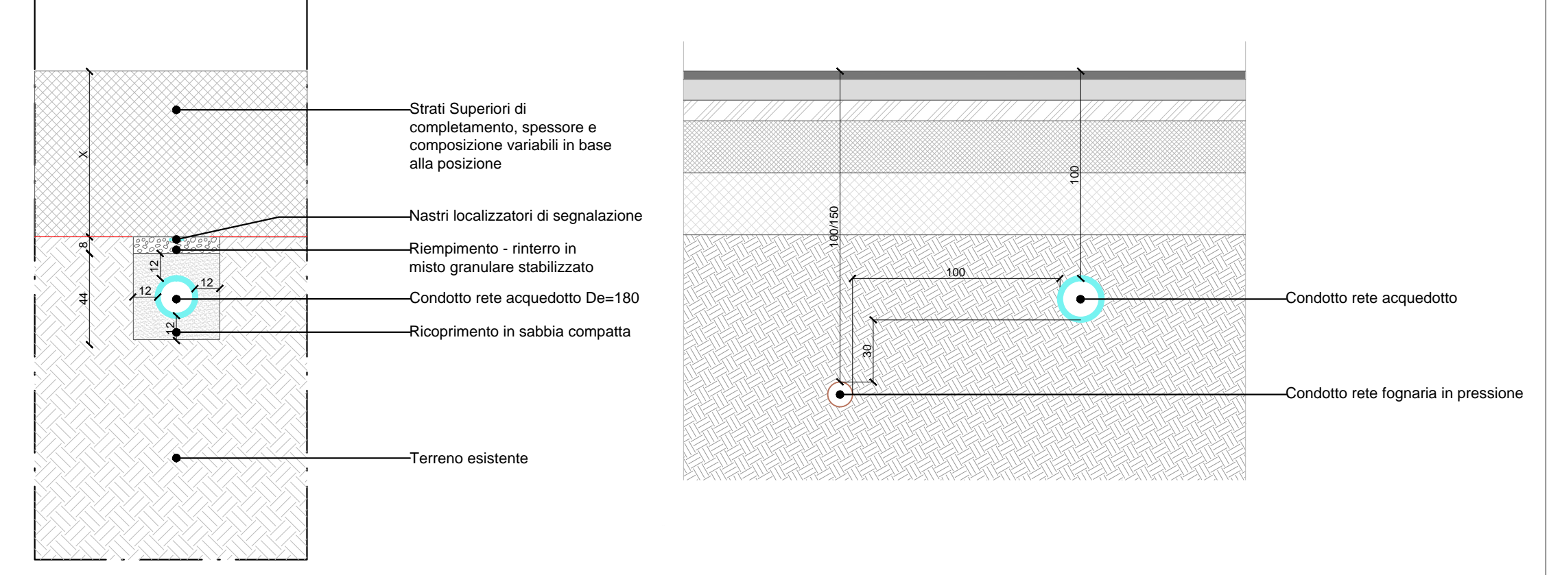
Dettaglio costruttivo rete idrica (scala 1:20)
