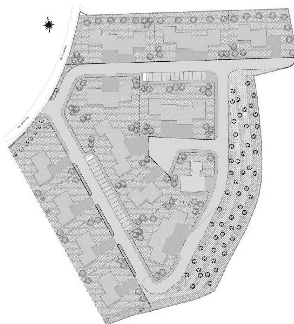
Planivolumetrico dell'intervento
