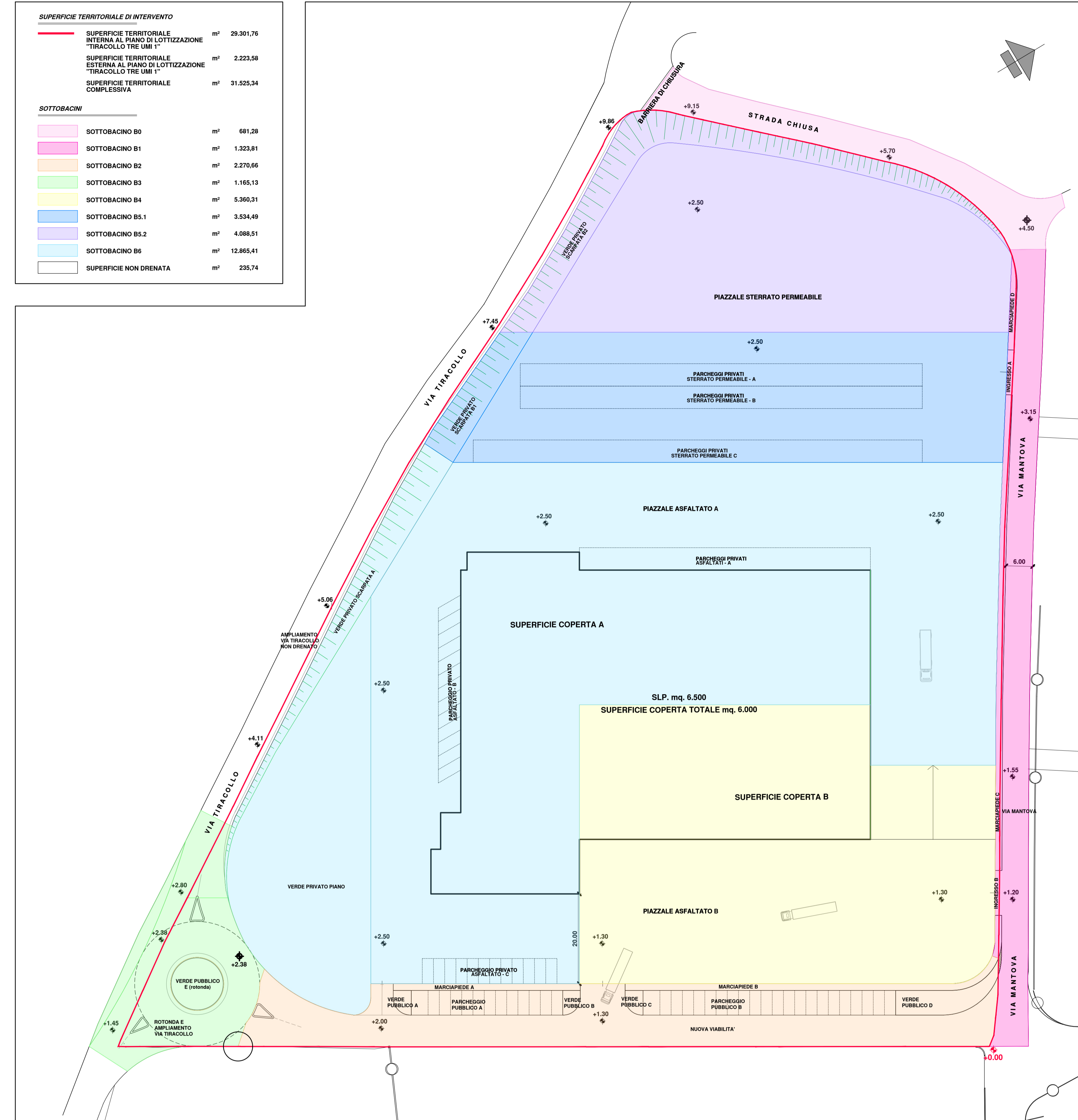
PLANIMETRIA SOTTOBACINI DI CALCOLO scala 1:500
