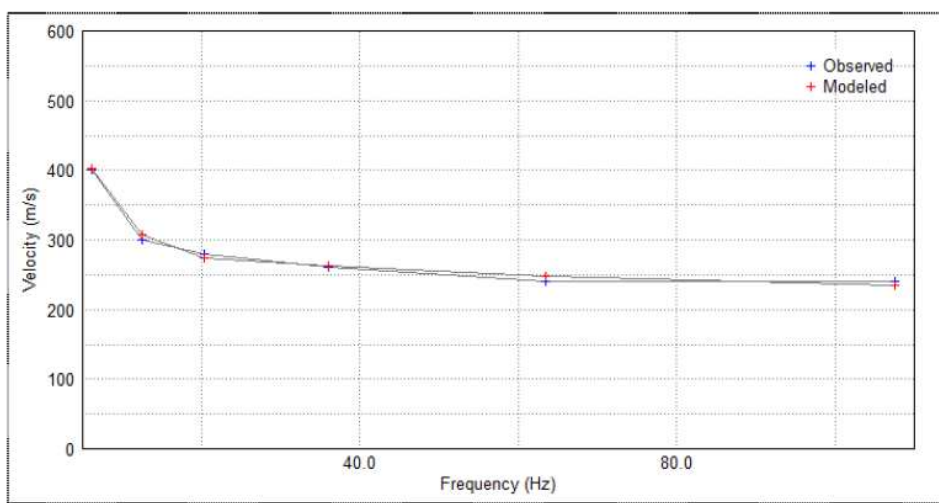
Fig. n.24 – Curva di dispersione sperimentale osservata e derivante dal modello
