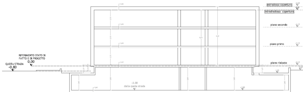
Fig. n.9 – Sezione AA' STATO DI PROGETTO Scala 1:250
