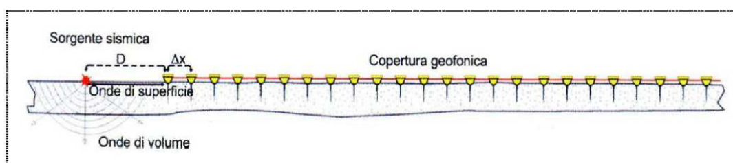
Fig. n.20 - Disposizione geometrica di una prova MASW
