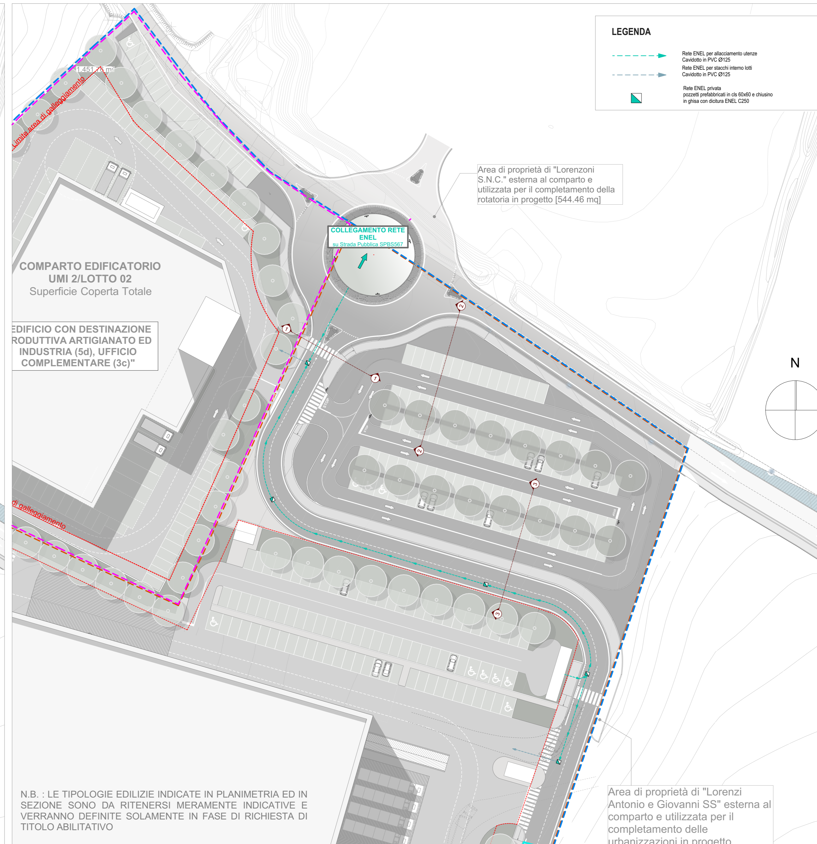
PLANIMETRIA GENERALE con individuazione RETE ENEL PRIVATA Scala 1:500
