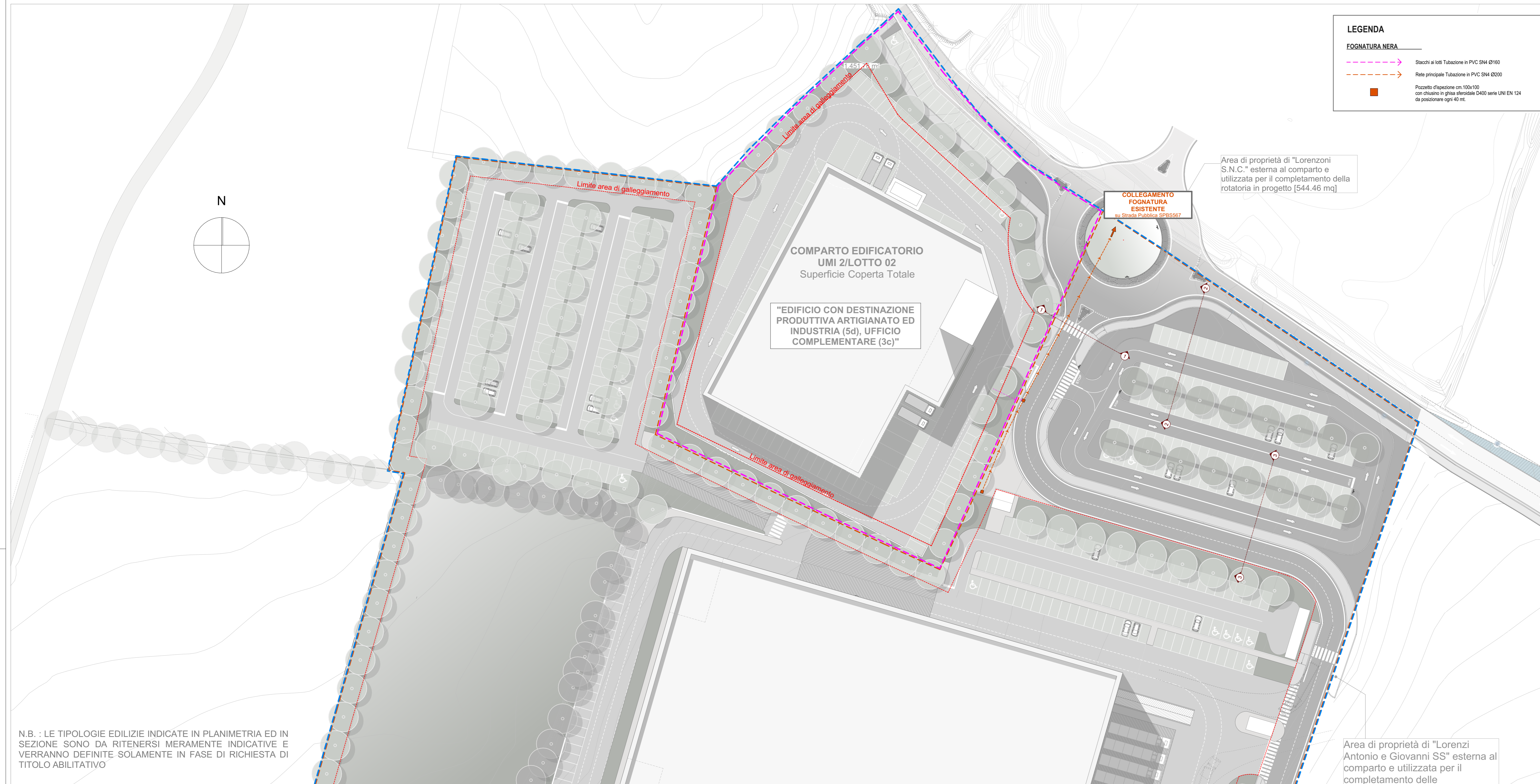
PLANIMETRIA GENERALE con individuazione RETI ACQUE NERE Scala 1:500
