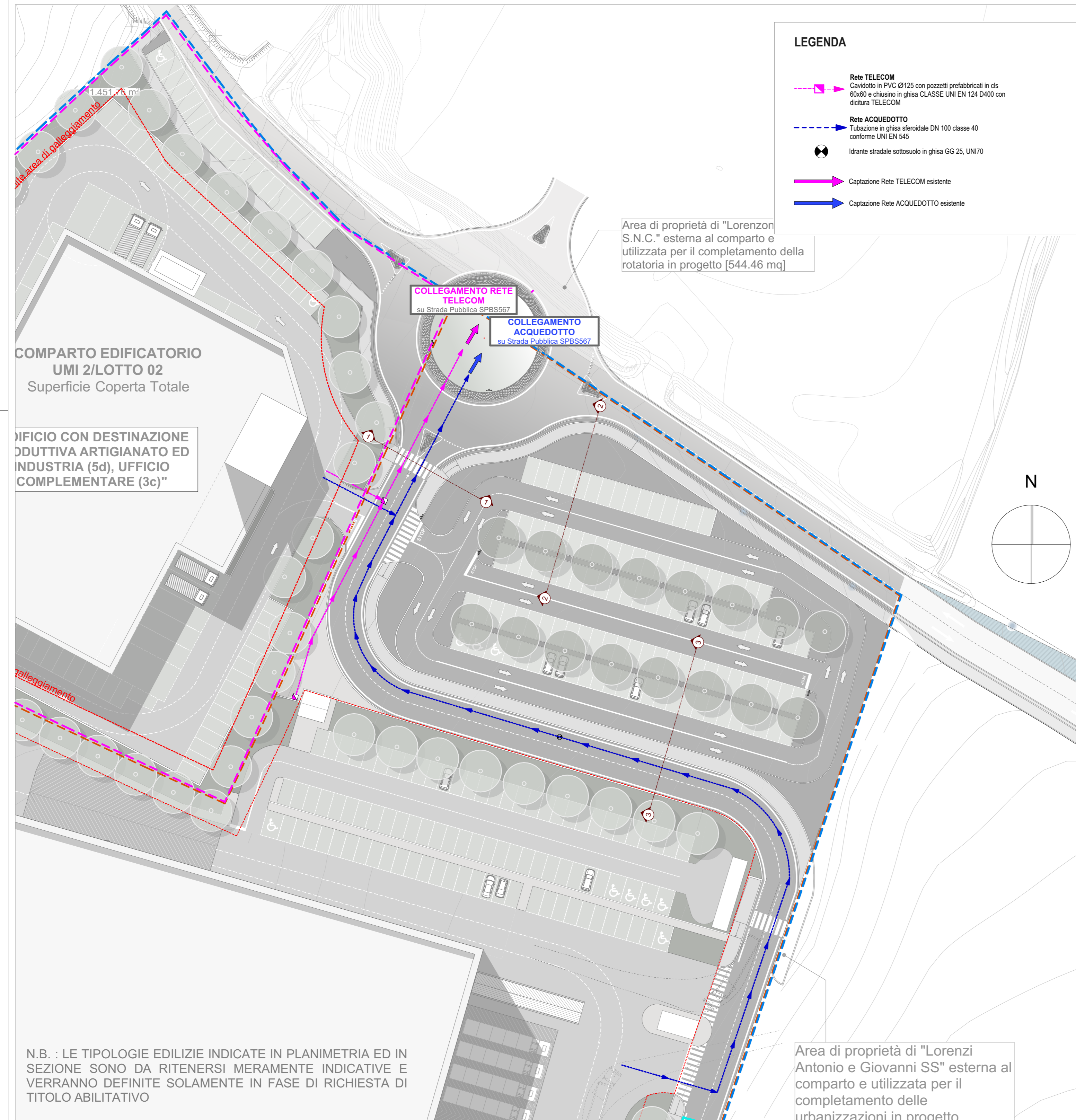
PLANIMETRIA GENERALE con individuazione RETI TELECOM - ACQUEDOTTO Scala 1:500
